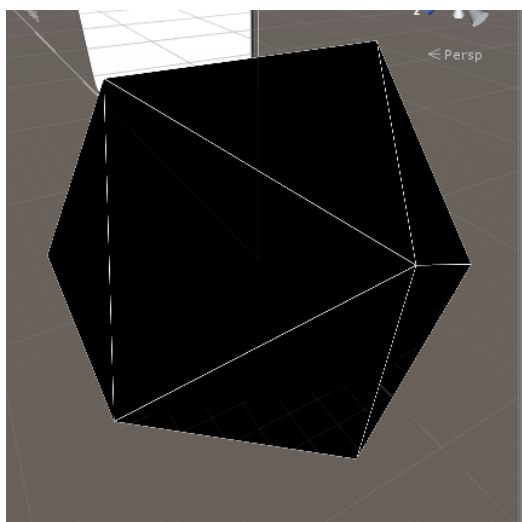
Slika 36: Wireframe ikosaedar
