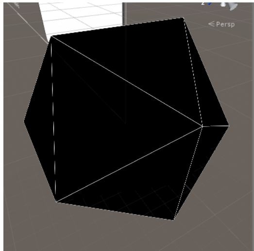
Slika 36: Wireframe ikosaedar
