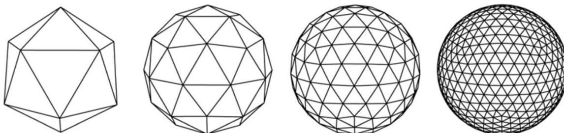
Slika 5: Ikozaedrena sfera [13]
