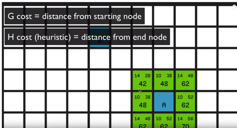
Grafički prikaz načina na koji radi A* algoritam [5]
