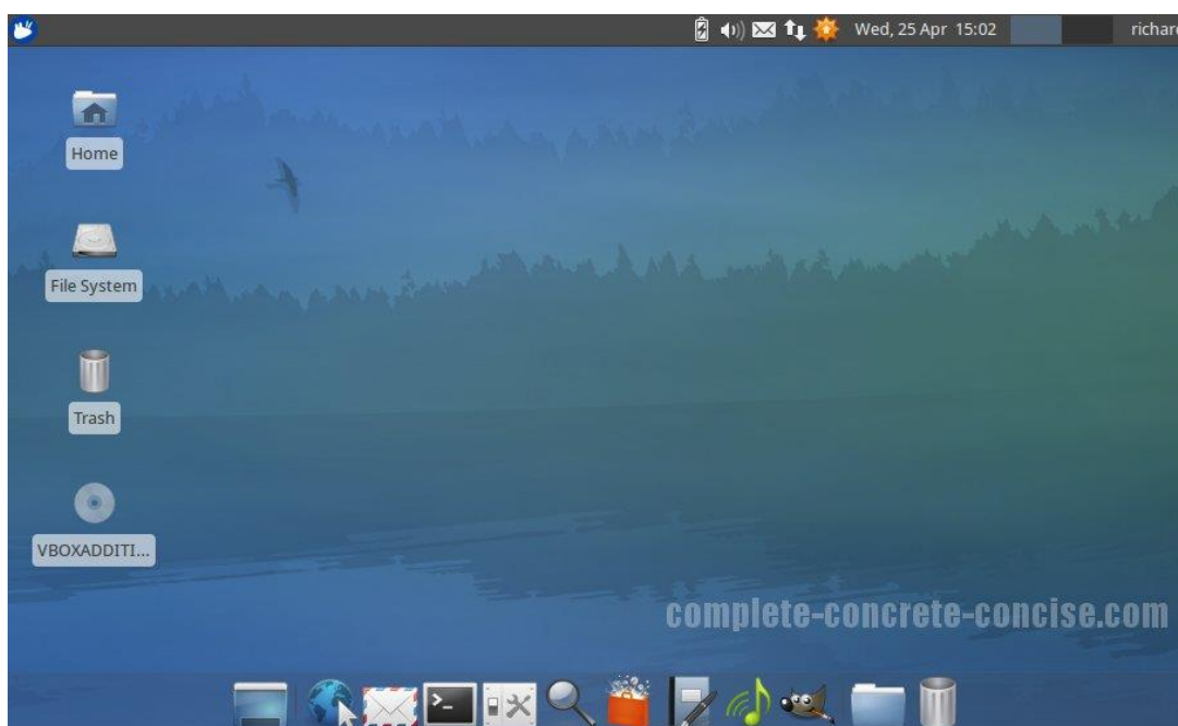
Slika 6. Xubuntu desktop
