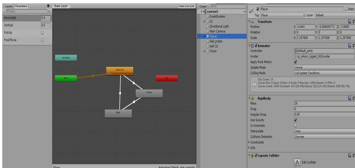
Slika 21 Animator Controller
