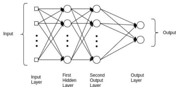
Slika 3: Višeslojni perceptron [15]
