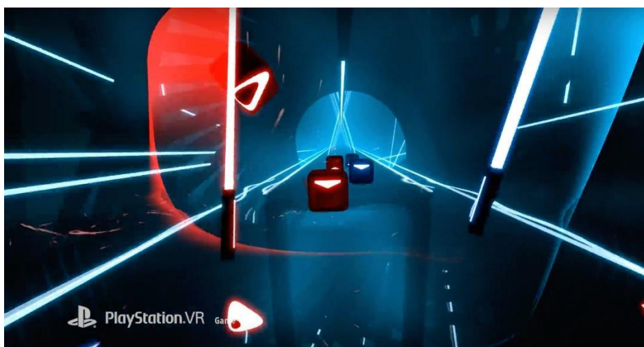
Slika 8 Beat Saber
