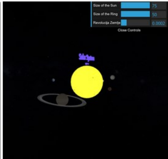
Slika 34: Sunčev sustav
