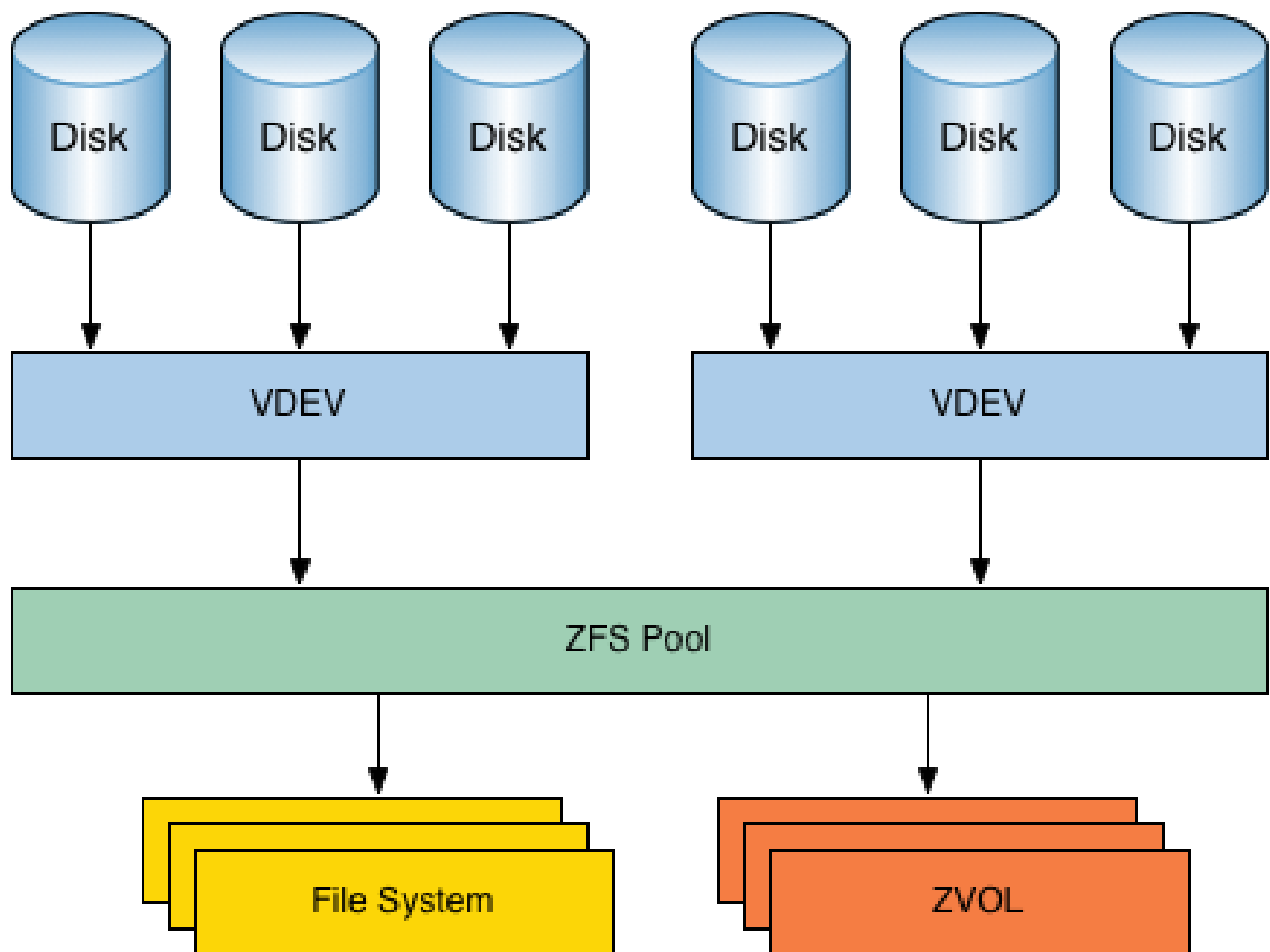
Slika 6: Arhitektura ZFS-a [26]
