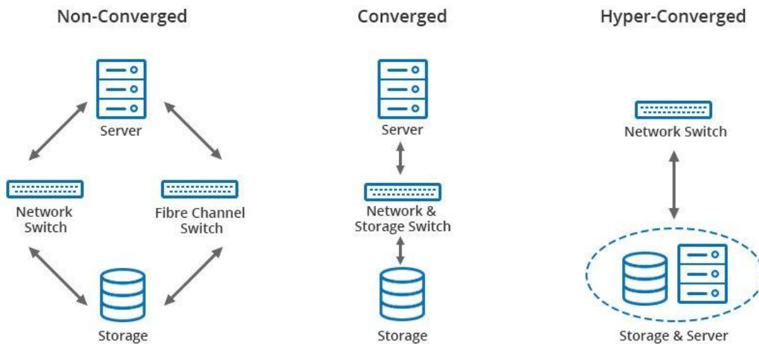
Slika 2: Usporedba infrastruktura [20]
