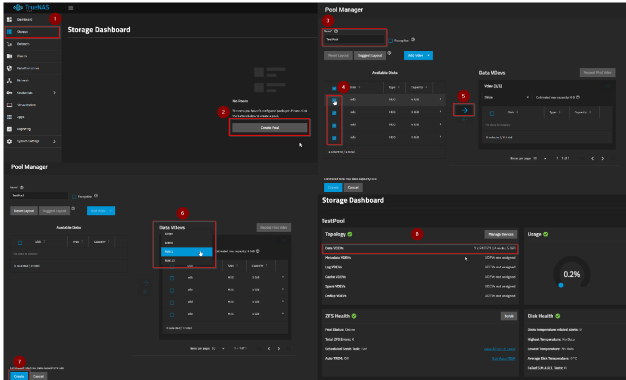
Slika 7: Konfiguracija ZFS-a
