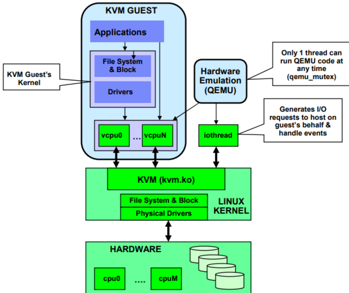
Slika 12: Arhitektura KVM-a [41]
