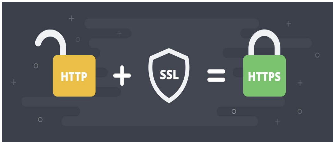
Slika 13. HTTPS protokol
