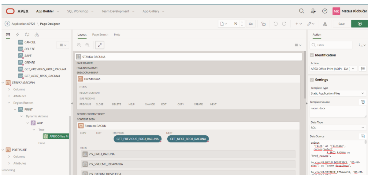
Slika 57. Izrada ispisa računa u Dizajneru stranice
