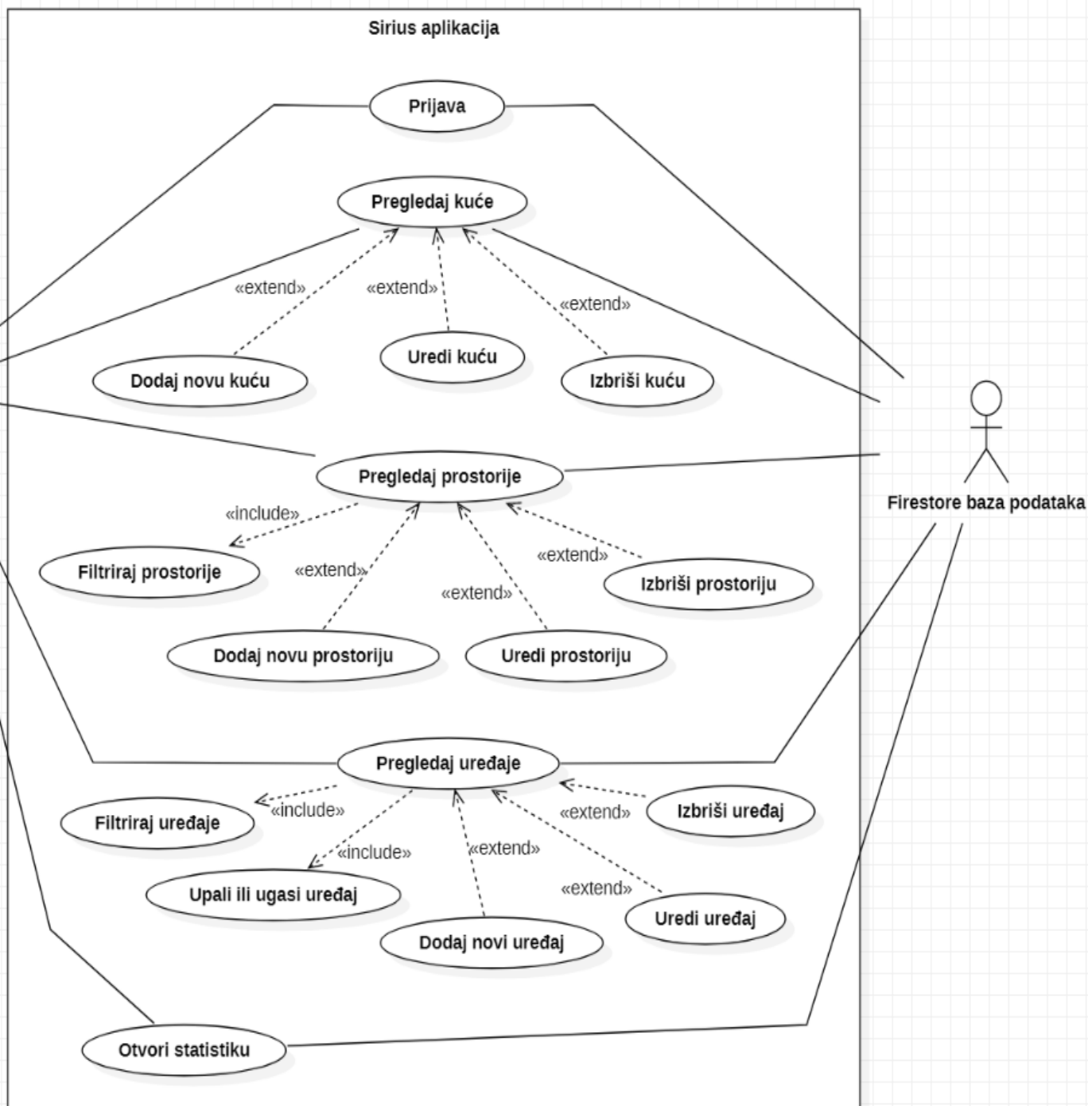
Slika 4 - use case dijagram za Sirius aplikaciju
