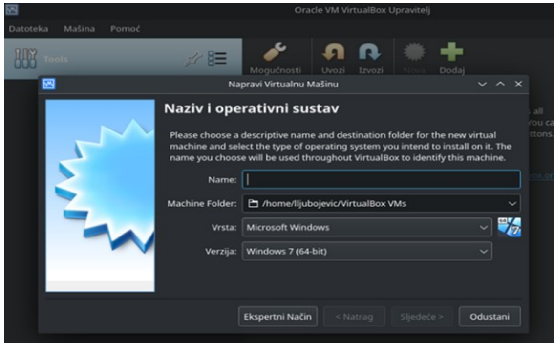
Slika 15: Oracle VirtualBox
