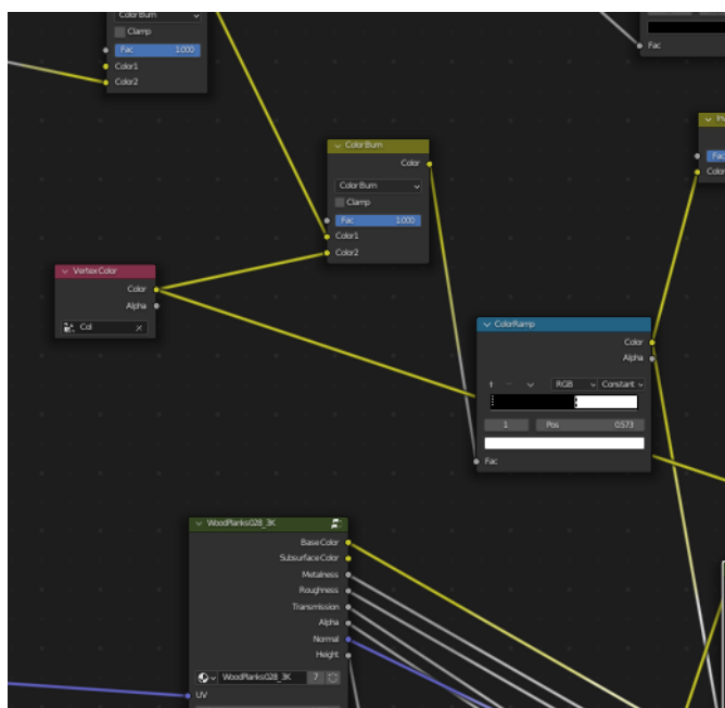
Slika 36. Vertex Color
