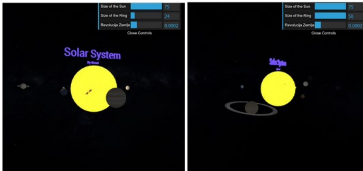
Slika 34: Sunčev sustav
