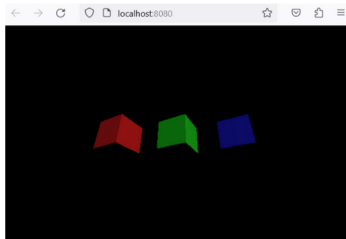
Slika 9: Usmjereno svjetlo
