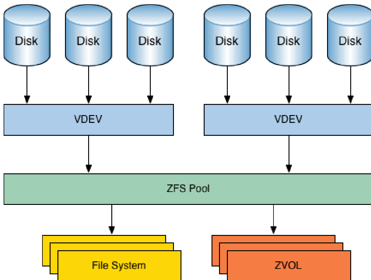
Slika 6: Arhitektura ZFS-a [26]
