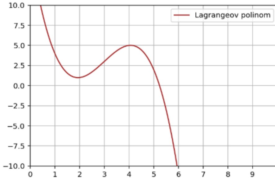
Slika 9. Lagrangeov polinom
