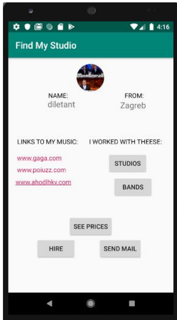
Slika 13. Aktivnost VisitProfile
