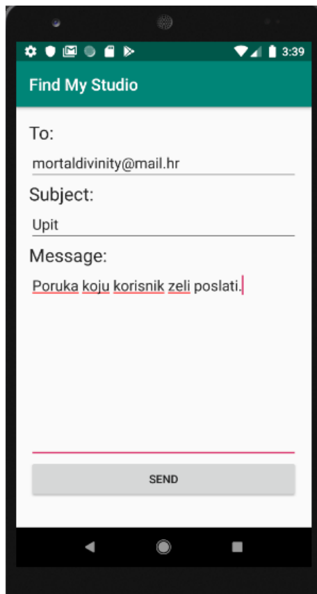
Slika 14. Aktivnost SendMail
