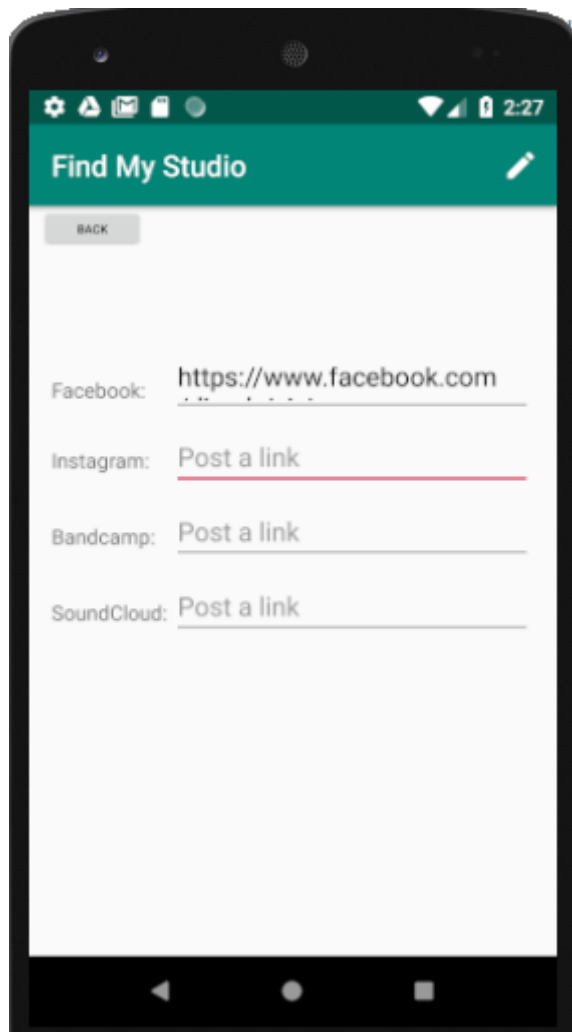
Slika 10. Aktivnost UpdateLinks
