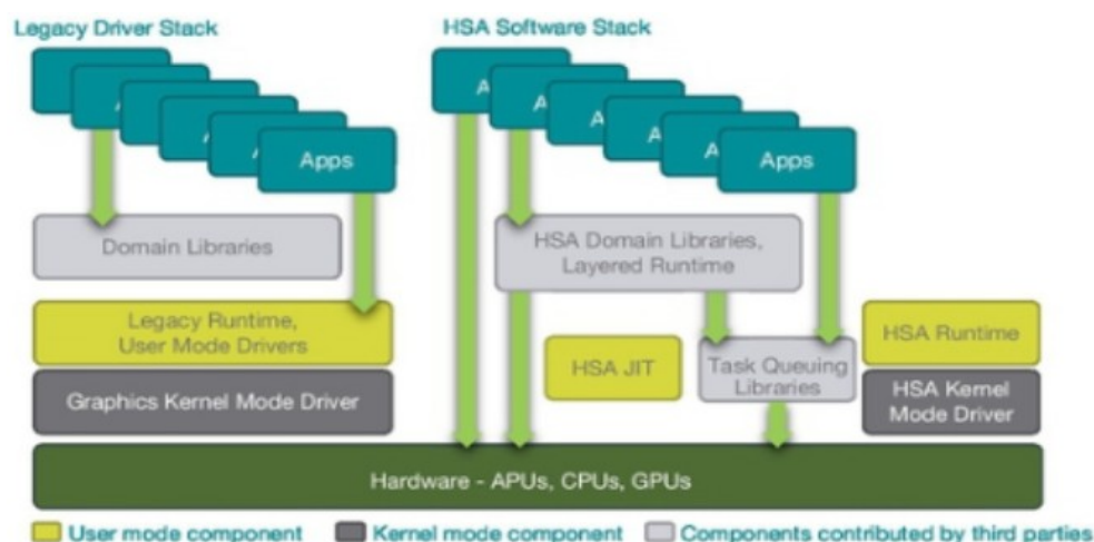
Slika 5: Izvođenje HSA softvera. [30]
