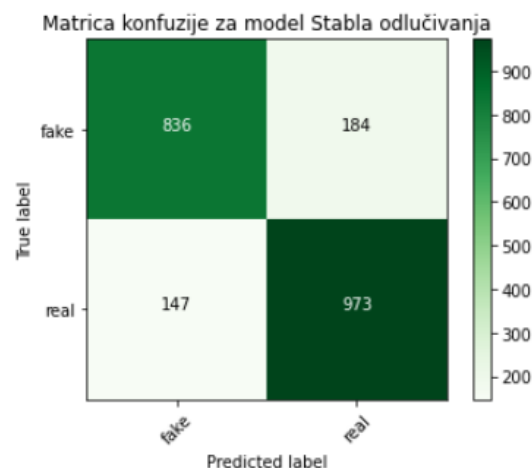
Slika 37. Rezultati za stablo odlučivanja
