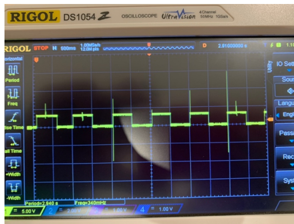
Slika 9 - Osciloskopsko mjerenje elektromagnetskih smetnji - šire
