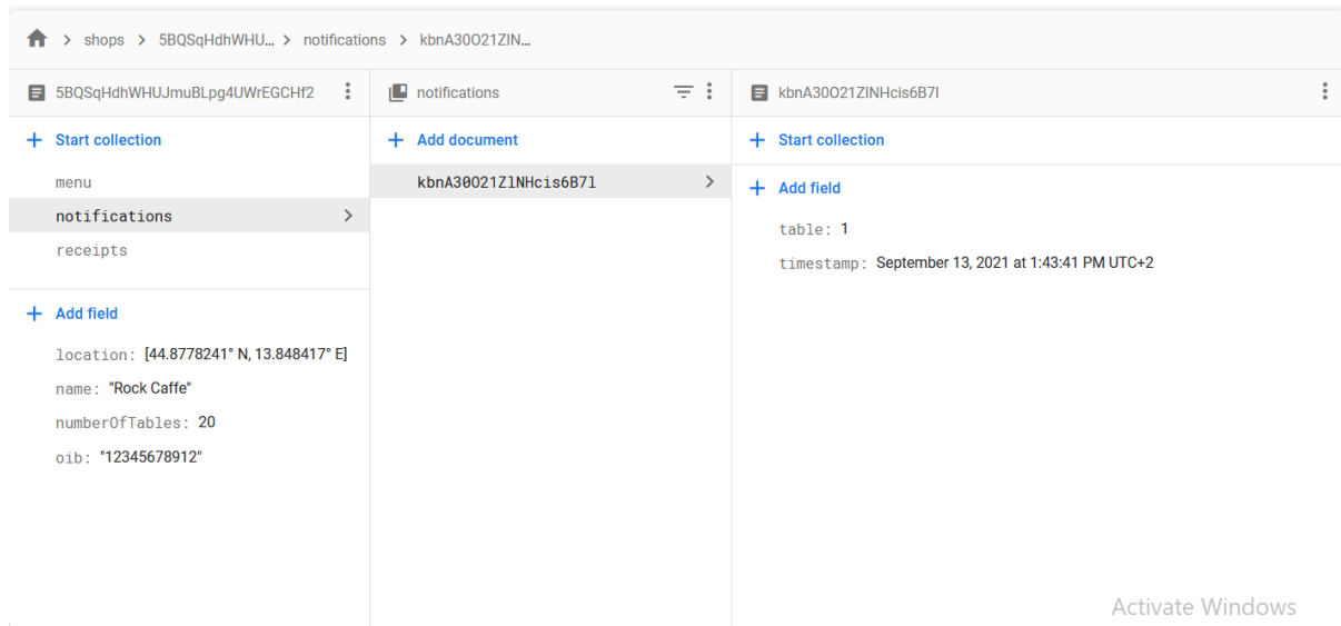
Slika 9: Podkolekcija notifications
